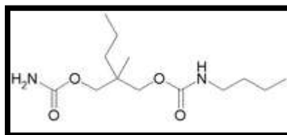
Fig. Tybamate.
