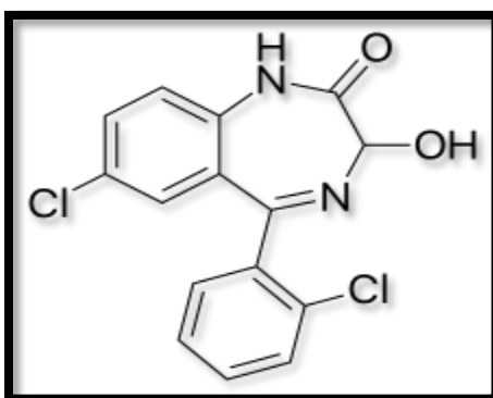
Fig. Lorazepam.
